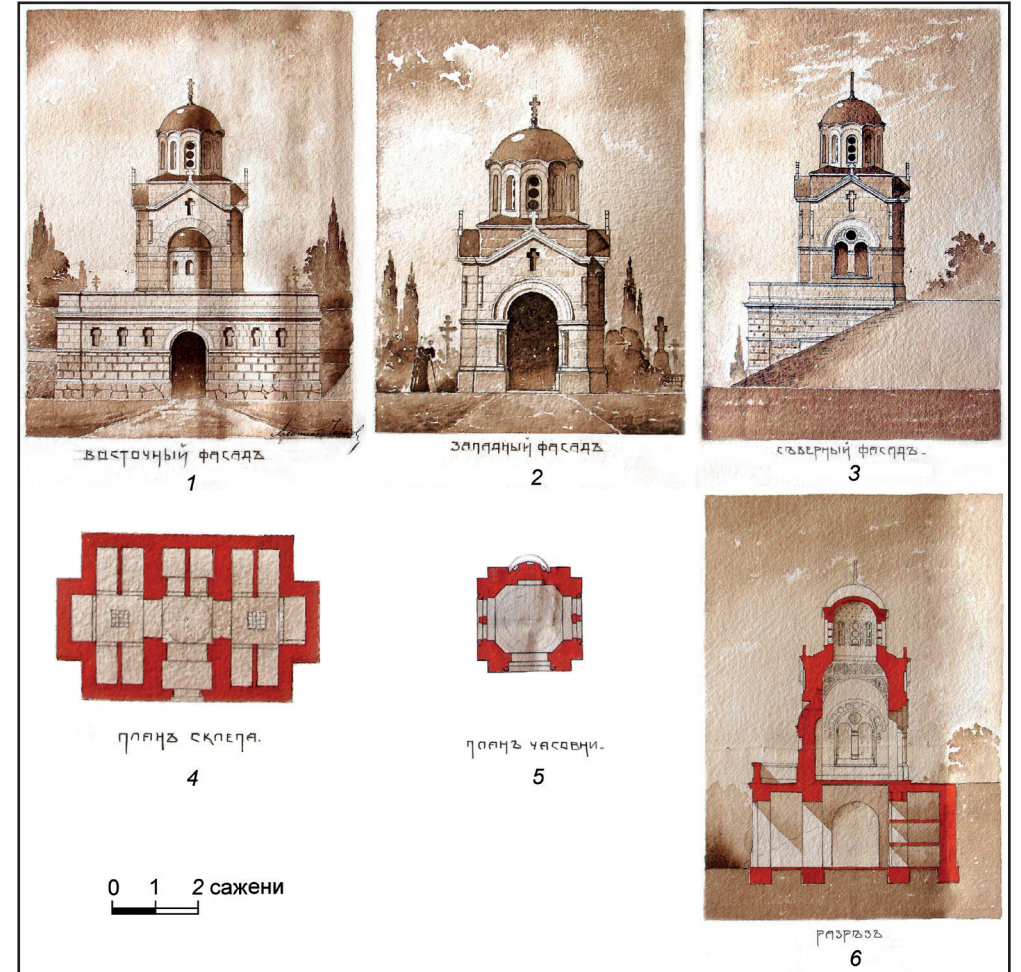
Проект здания Михайловской часовни. Архитектор В. А. Чистов. 1912 г. ГАРК
